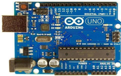
Fig.4.3.1: Arduino Microcontroller
